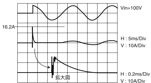
AC.100V系 サージ電流
