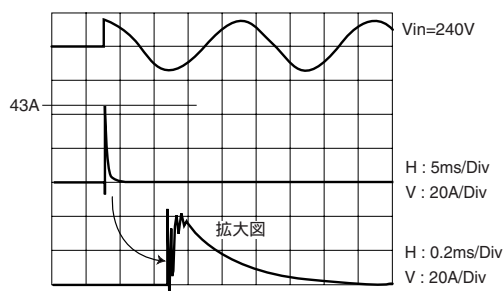
AC.200V系 サージ電流
